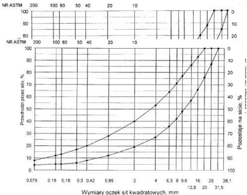
Rys.1. Krzywe graniczne uziarnienia mieszanki mineralnej BA od 0 do 31,5 mm do podbudowy nawierzchni drogi o obciążeniu ruchem KR 1 lub KR 2
