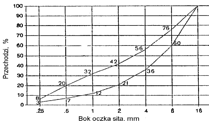
Rysunek 1. Krzywe graniczne uziarnienia kruszywa do betonu
